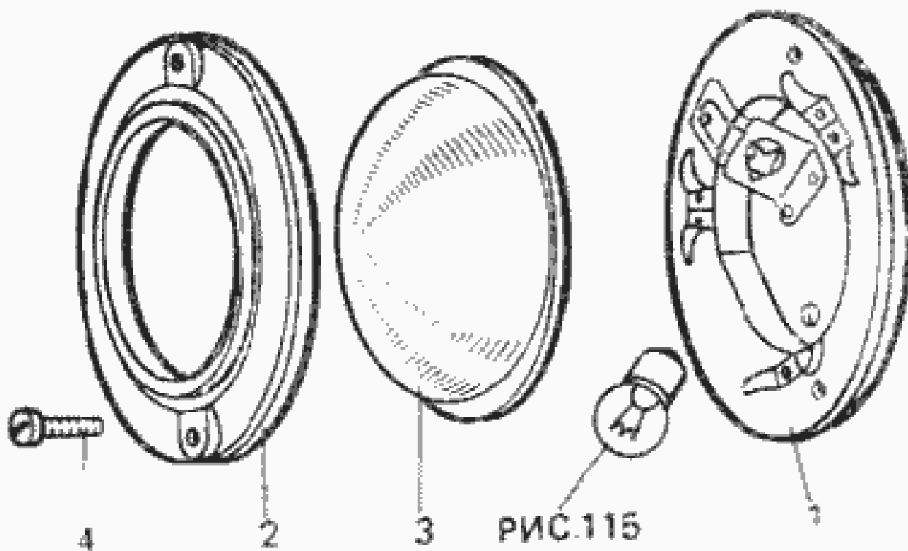
Рис. 119. Плафон ПК201-3714010-Д
